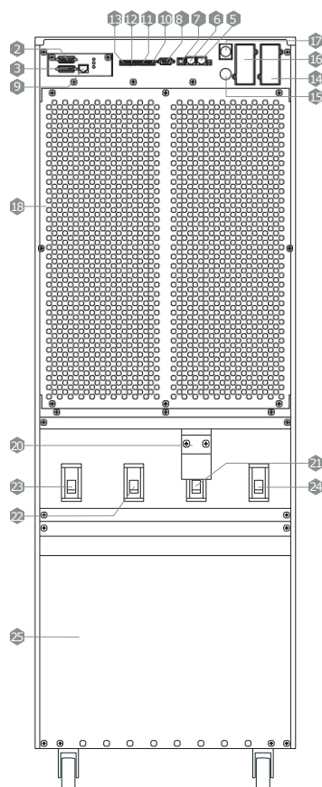
Вид сзади: КС33160Н (160кВА)
