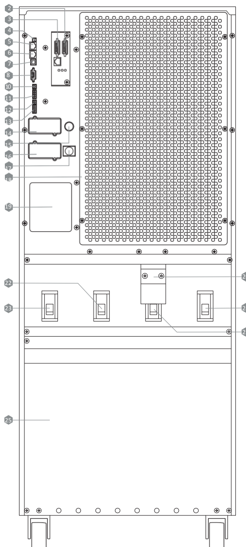
Вид сзади: KC3380H (80 кВА); KC33100H (100 кВА); KC33120H (120 кВА)
