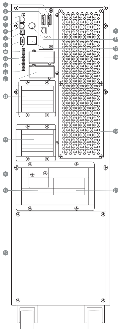
Вид сзади: KC3360H (60 кВА)
