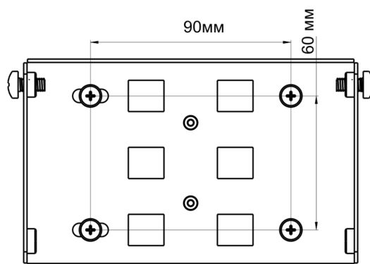
Рисунок 12 – Расстояния между отверстиями крепления
