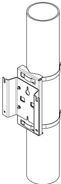
Рисунок 8 – Крепление кронштейна на трубостойку
