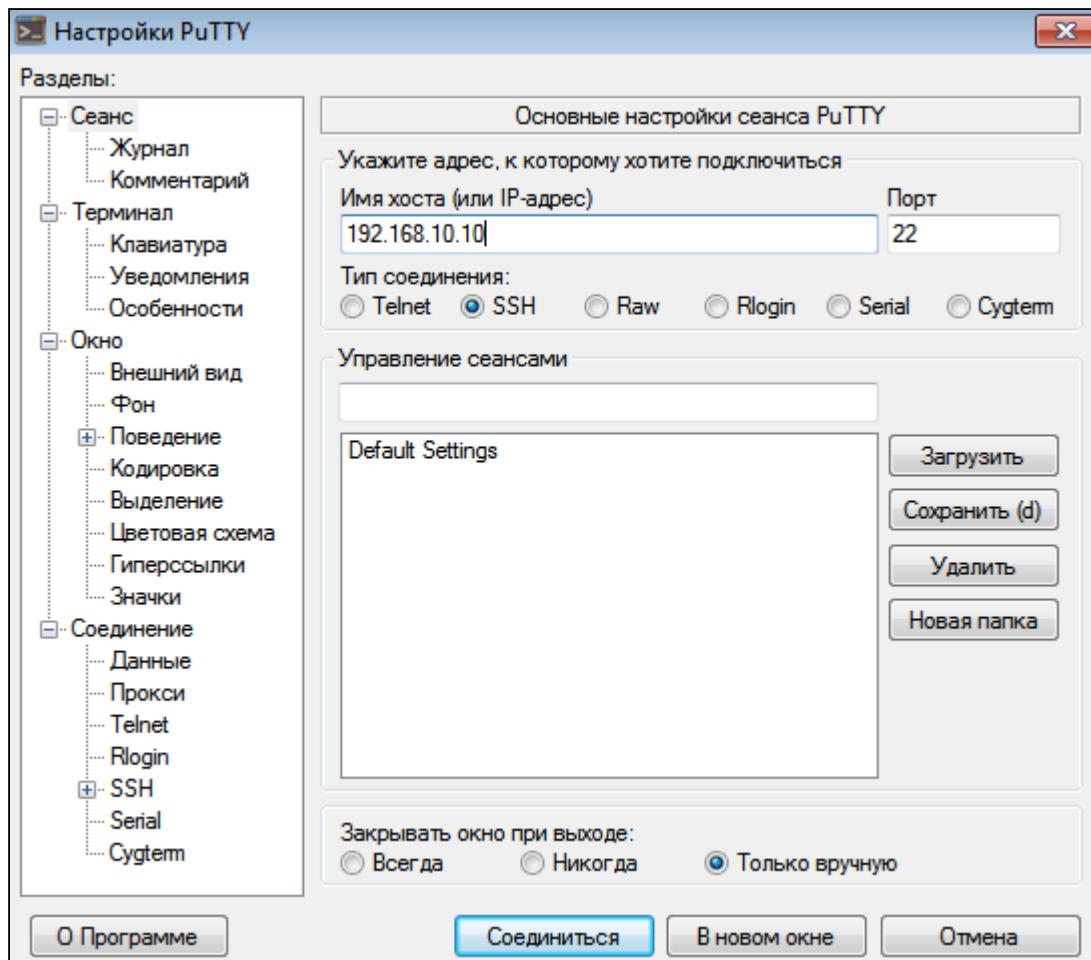
Рисунок 35 – Запуск SSH-клиента
