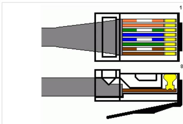
Рисунок 20 – Разъем RJ-45
