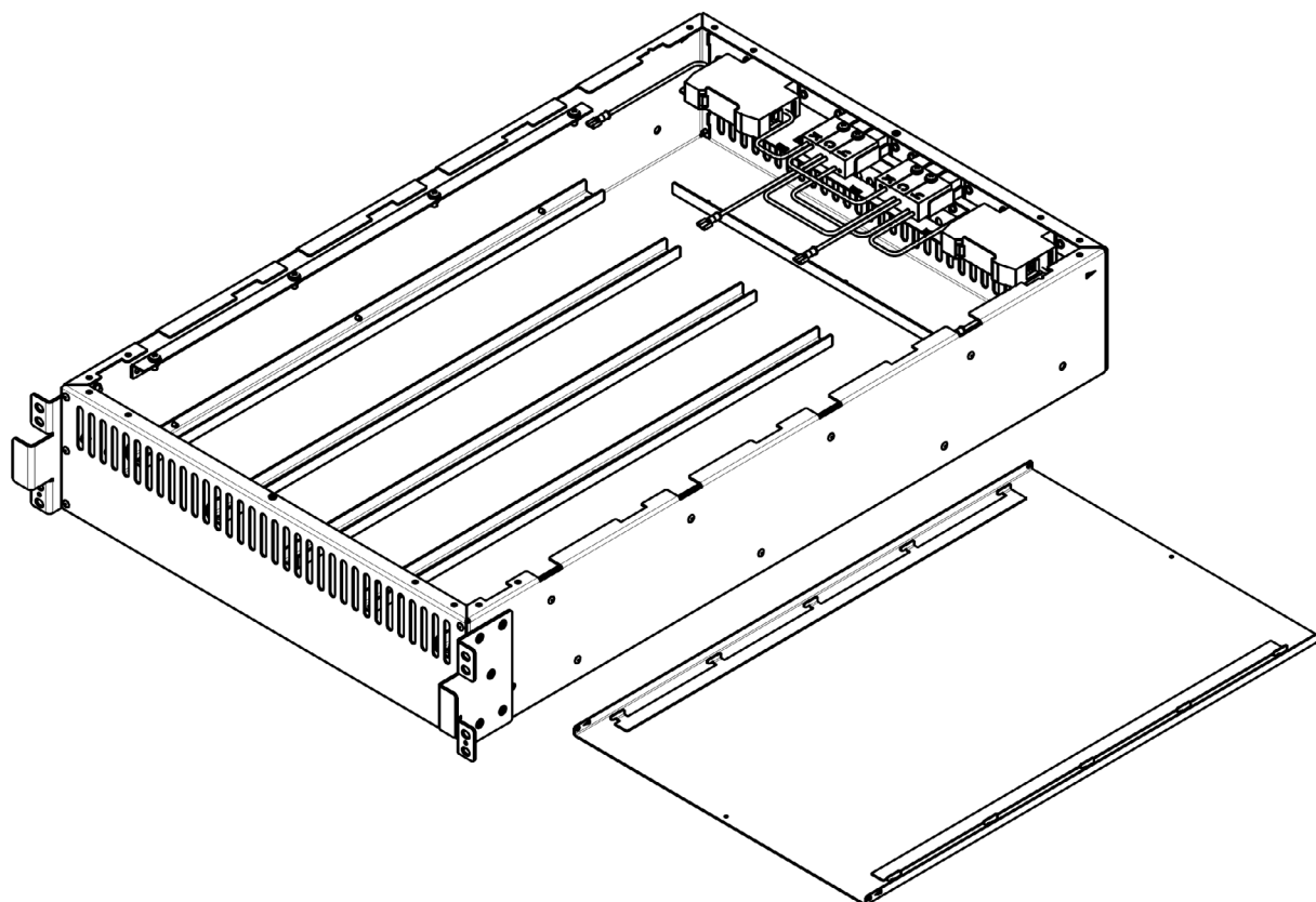
Рисунок 3 - Вид внутри
