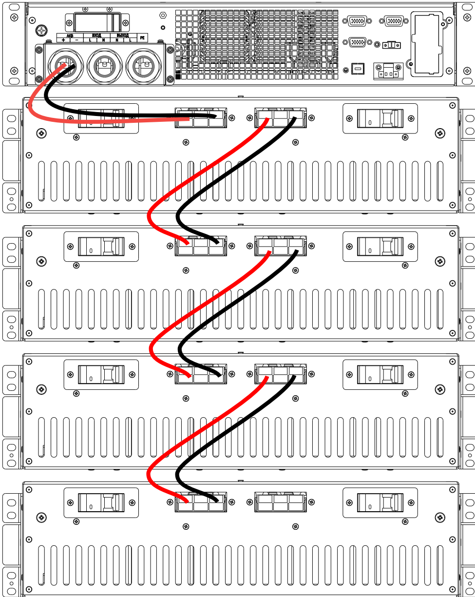
Рисунок 4 - Подключение батарейного модуля к ИБП
