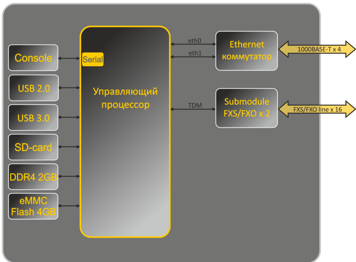
Рисунок 3 – Функциональная схема SMG-200
