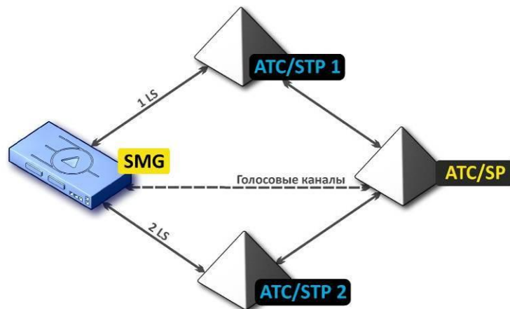
Рисунок 19 – Схема подключения SMG в комбинированном режиме
