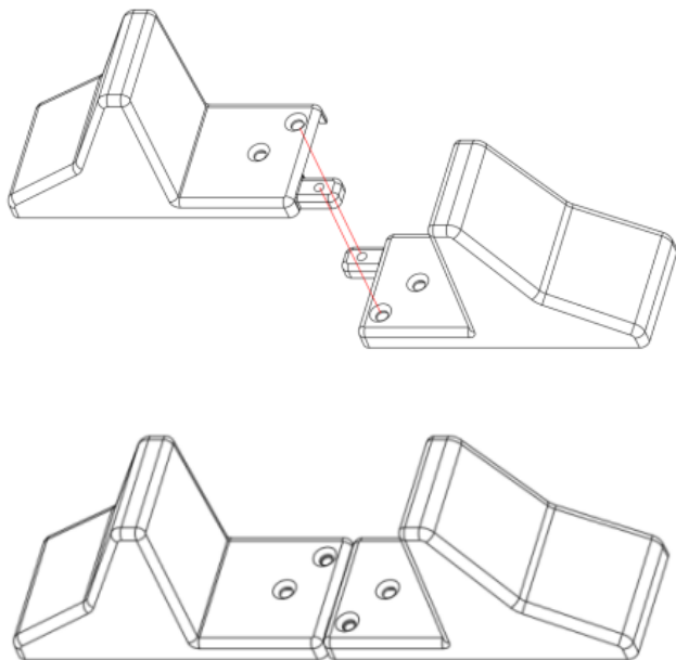
Рисунок 5-1 Сборка подставки для вертикальной установки
