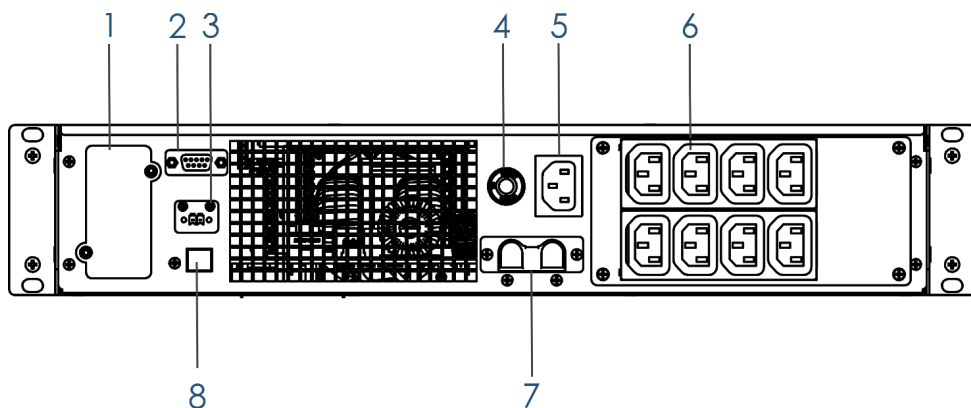
Рисунок 1-2 Вид сзади ИБП 1 кВА
