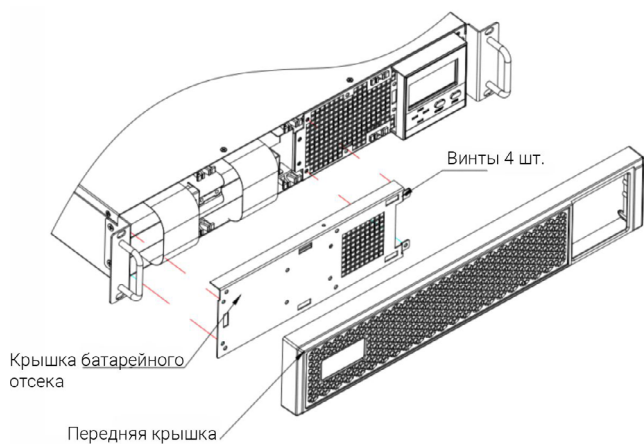
Рисунок 8-1 Снятие фронтальной панели и крышки батарейного отсека
