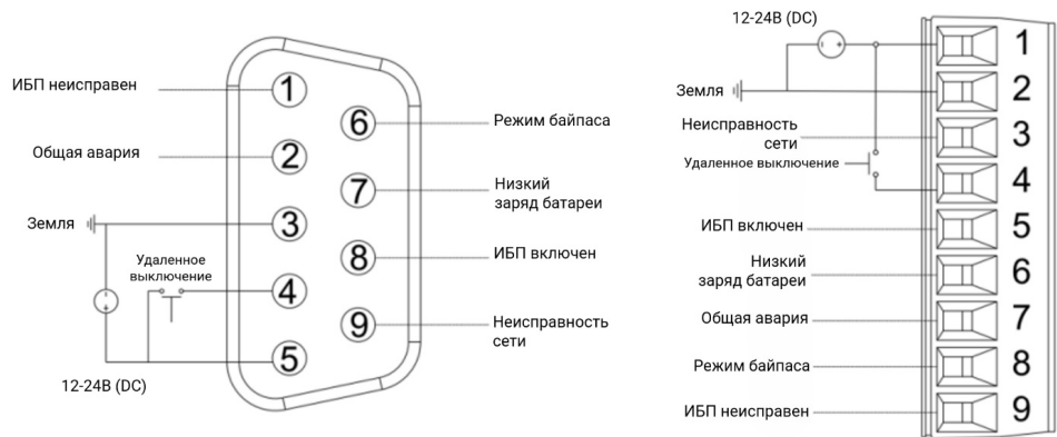
Рисунок 8 – Схема подключения сухих контактов
