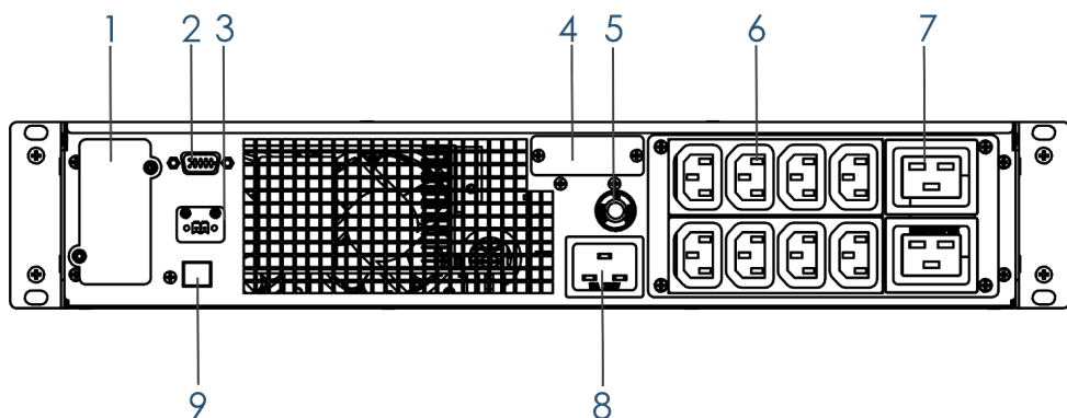
Рисунок 1-3 Вид сзади ИБП 2-3 кВА
