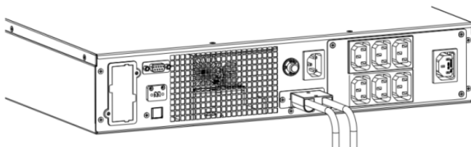
Рисунок 5-6 Подключение батарейного разъема
