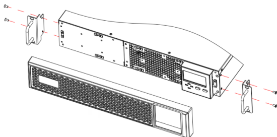
Рисунок 5-2 Снятие передней панели
