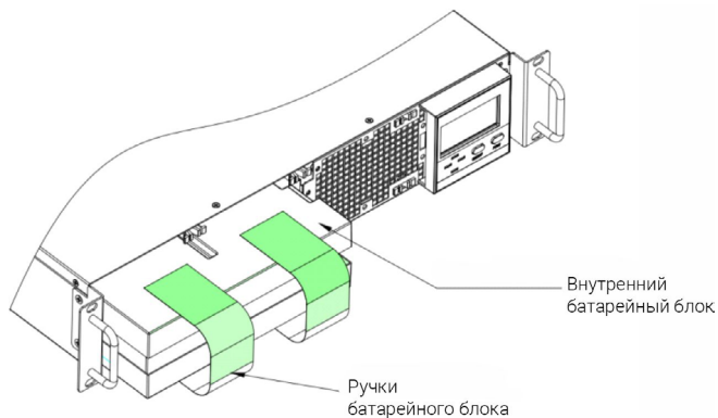
Рисунок 8-2 Извлечение внутреннего батарейного блока
