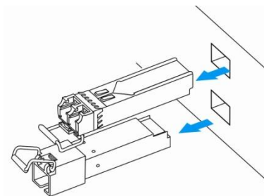
Рисунок 33 – Извлечение SFP-трансиверов
