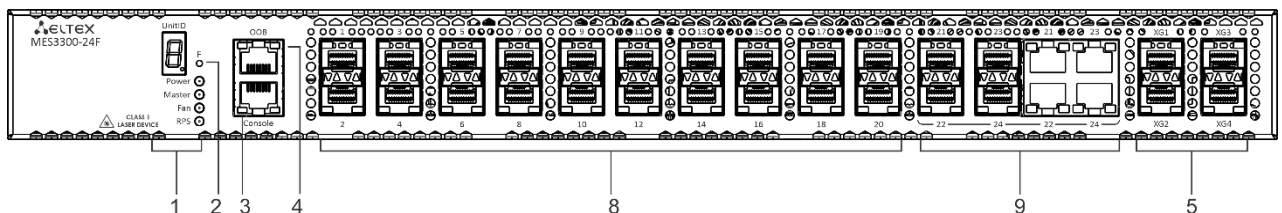
Рисунок 1 – Передняя панель MES3300-24F
