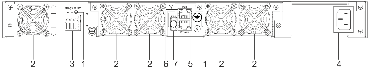
Рисунок 12 – Задняя панель MES5400-48
