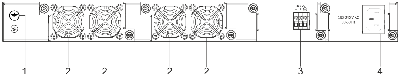
Рисунок 11 – Задняя панель MES5400-24
