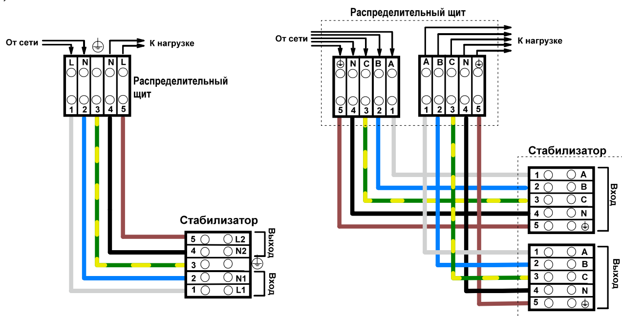
1- фазная сеть (используется 1 монтажный провод)
