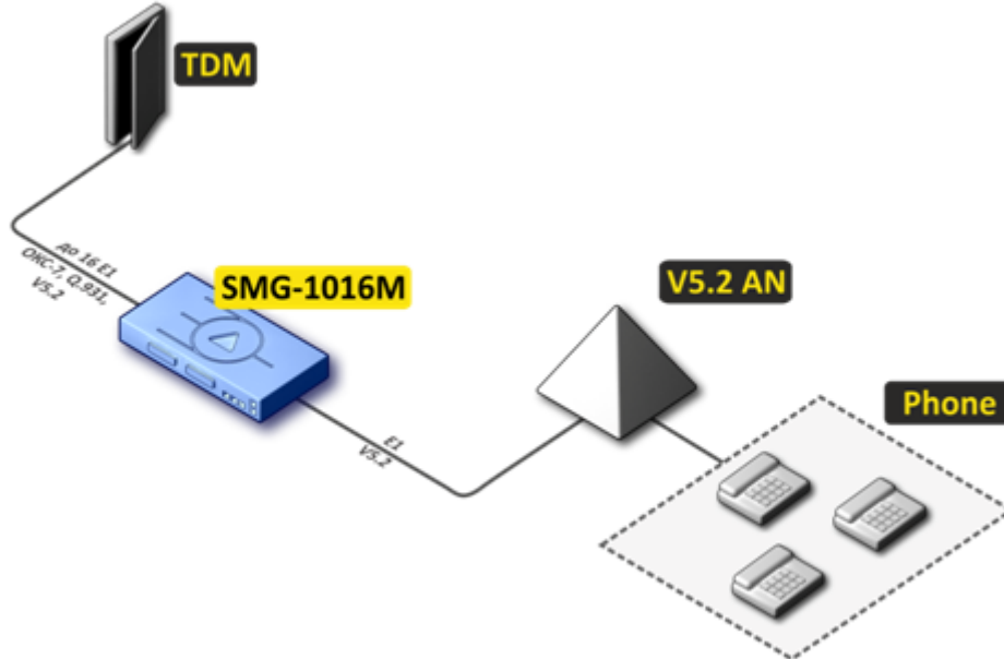
Рисунок 6 – Вынос V5.2 AN на базе SMG-1016M
