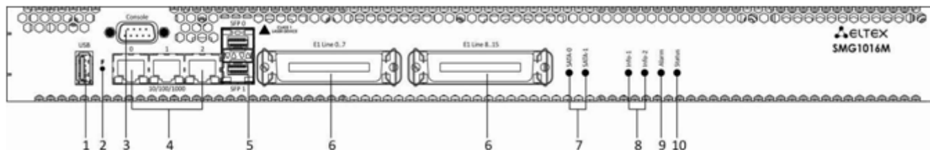
Рисунок 13 – Внешний вид передней панели SMG-1016M
