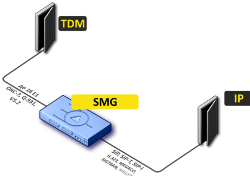
Рисунок 1 – Сопряжение сигнализаций и медиапотоков TDM- и VoIP-сетей
