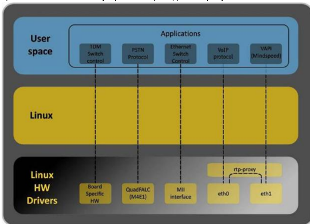
Рисунок 12 – Структура программного обеспечения SMG
