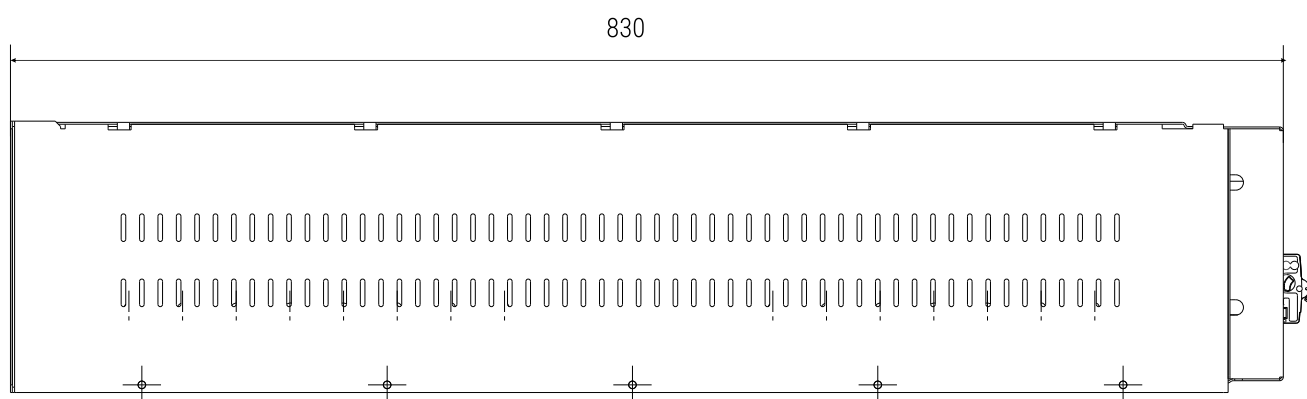
Внешний вид и габаритные размеры батарейного модуля DBR480S1
