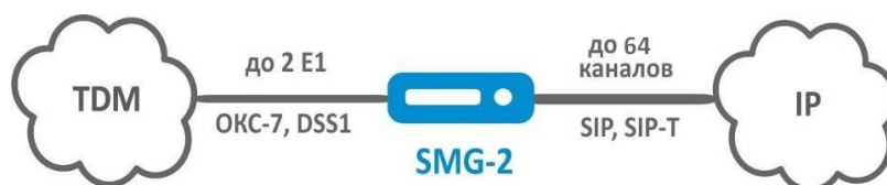
Рисунок 2 – Сопряжение сигнализаций и медиапотоків TDM- и VoIP-сетей с использованием SMG-2
