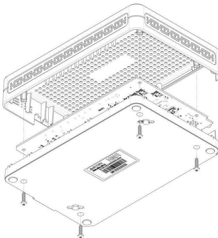
Рисунок 9 – Вскрытие корпуса
