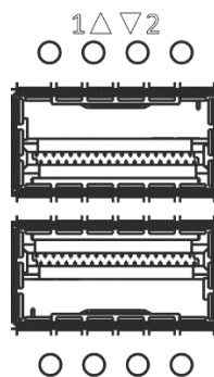
Рисунок 28 – Внешний вид разъема QSFP+ и QSFP28 для MES5500-32
