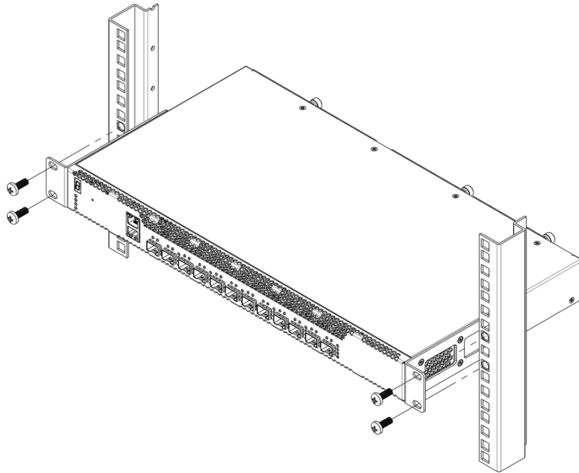
Рисунок 32 – Установка устройства в стойку
