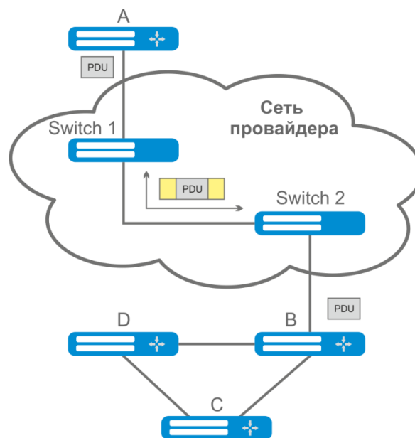
Рисунок 41 — Пример работы функции L2PT
