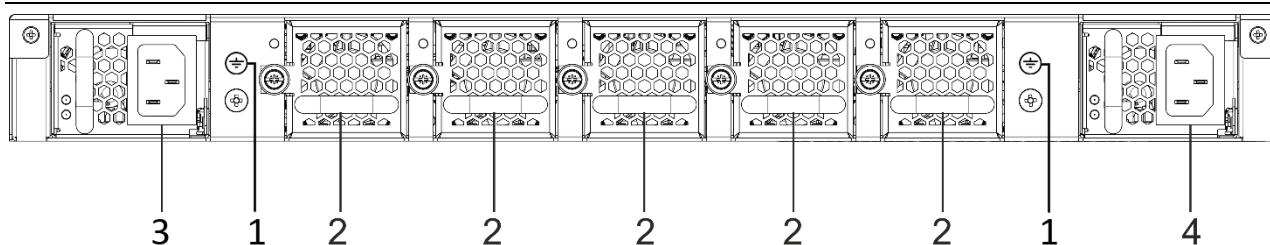
Рисунок 14 – Задняя панель MES5500-32
