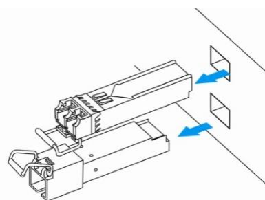
Рисунок 39 – Извлечение SFP-трансиверов
