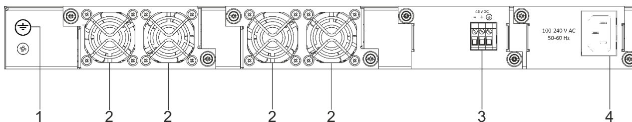
Рисунок 12 – Задняя панель MES5400-24
