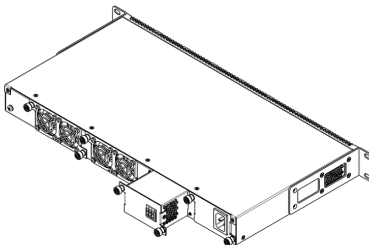
Рисунок 35 – Установка модулей питания
