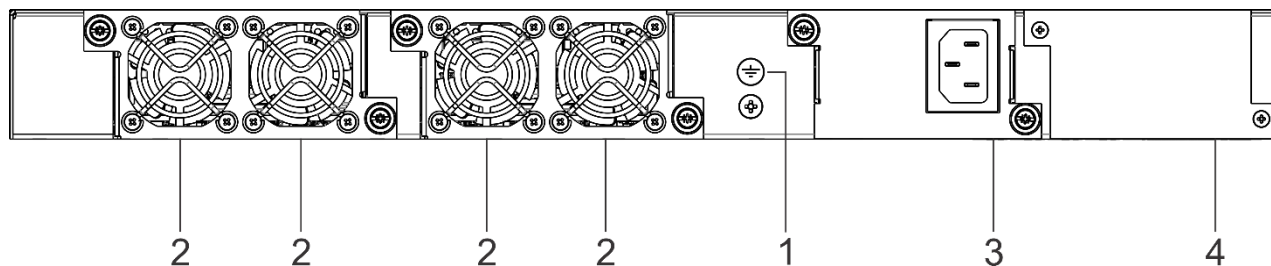
Рисунок 9 – Задняя панель MES3300-24F
