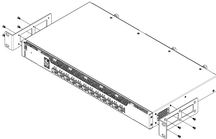
Рисунок 29 – Вариант крепления кронштейнов №1
