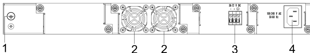
Рисунок 11 – Задняя панель MES5316A
