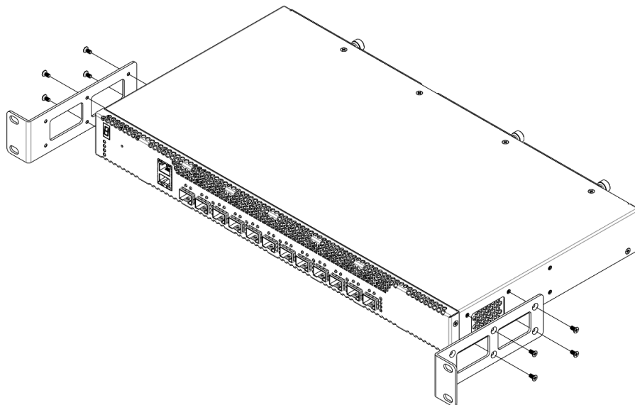
Рисунок 30 – Вариант крепления кронштейнов №2
