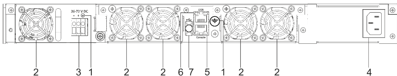
Рисунок 13 – Задняя панель MES5400-48
