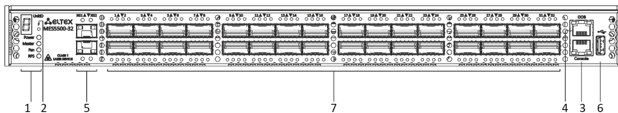
Рисунок 8 – Передняя панель MES5500-32
