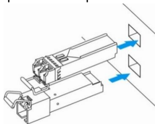
Рисунок 36 – Установка SFP-трансиверов
