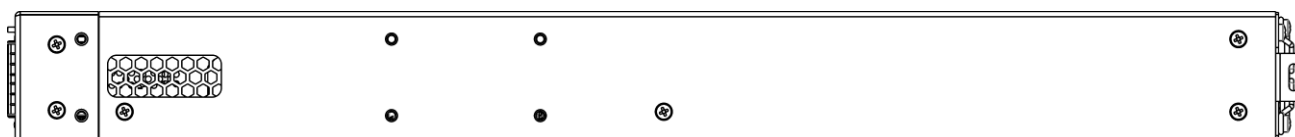
Рисунок 22 – Правая боковая панель Ethernet-коммутатора MES5400-48
