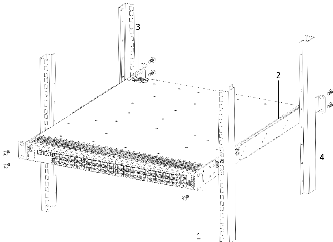
Рисунок 33 – Установка устройства MES5500-32 в стойку
