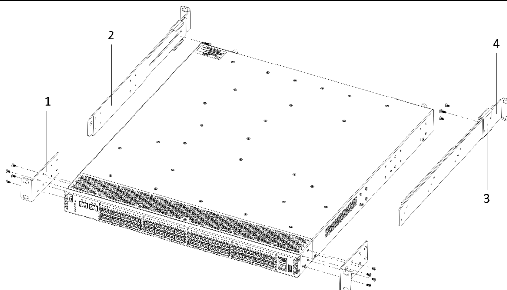
Рисунок 31 – Вариант крепления кронштейнов для MES5500-32
