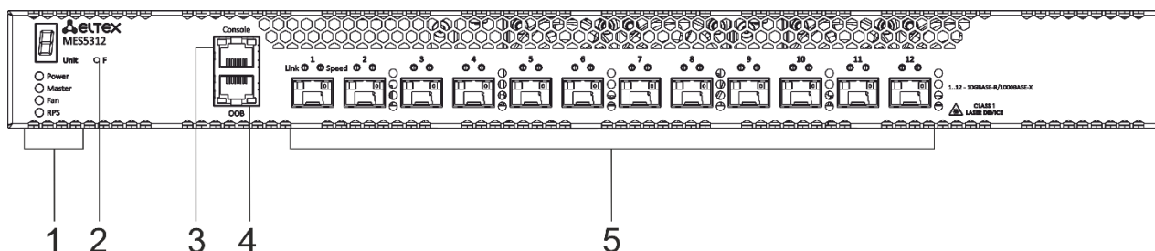
Рисунок 2 – Передняя панель MES5312
