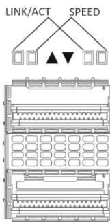
Рисунок 24 – Внешний вид разъема QSFP+ и QSFP28
