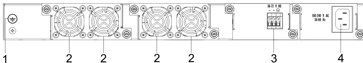
Рисунок 10 – Задняя панель MES5312, MES5324A, MES5332A
