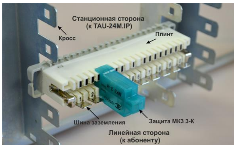
Рисунок 5 – Схема подключения
