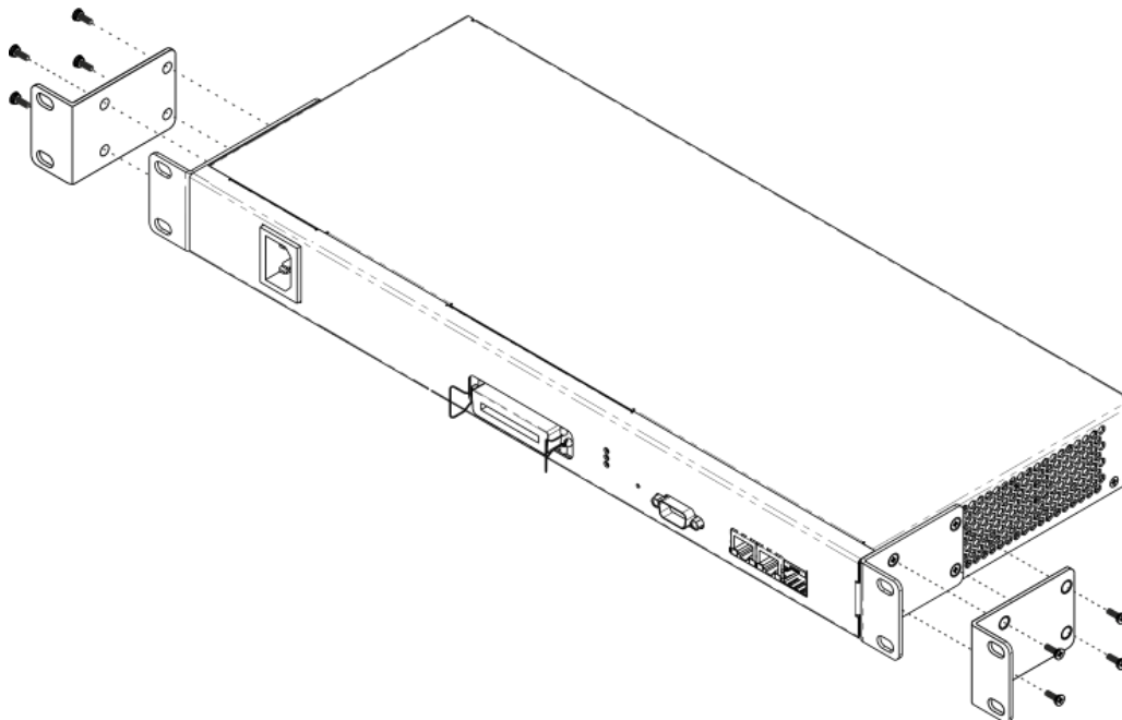
Рисунок 6 – Крепление кронштейнов
