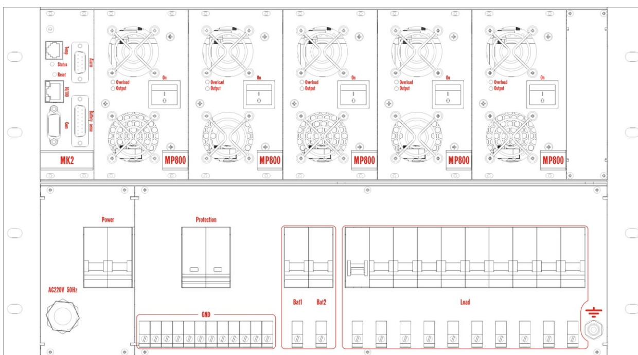
Рисунок 4 – Внешний вид УЭП2-5
