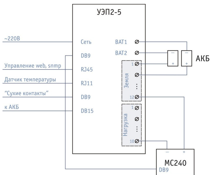
Рисунок 3 – Схема включения УЭП2-5
