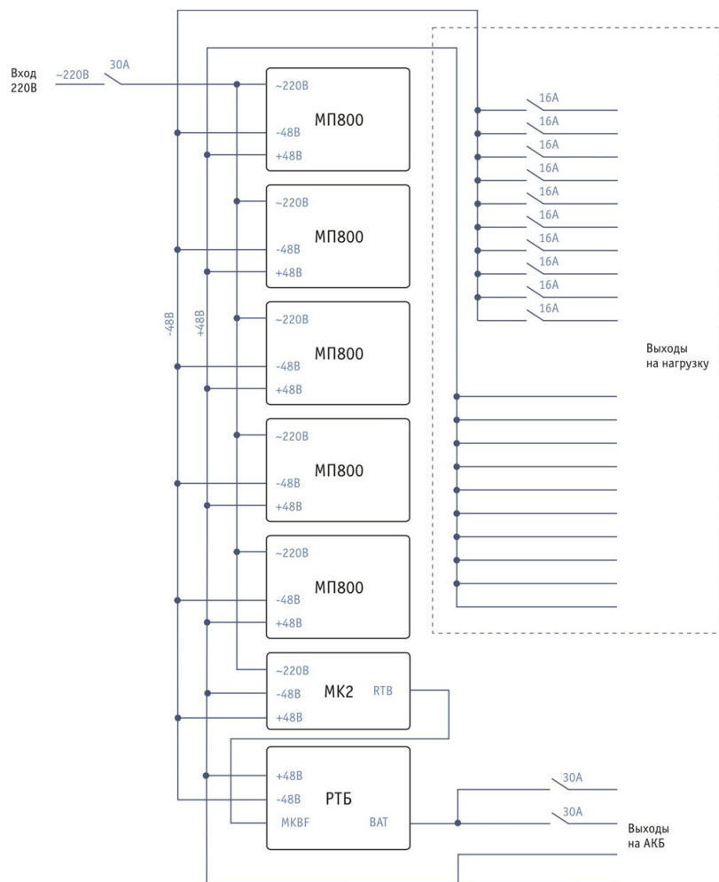
Рисунок 1 – Структурная схема устройства
