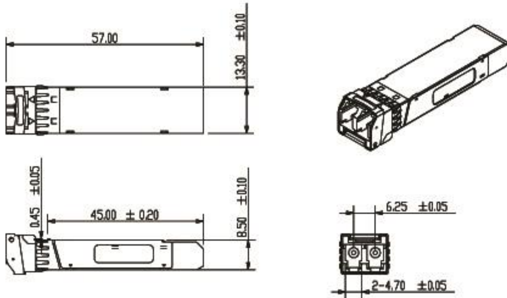
Рисунок 4. Механические характеристики
