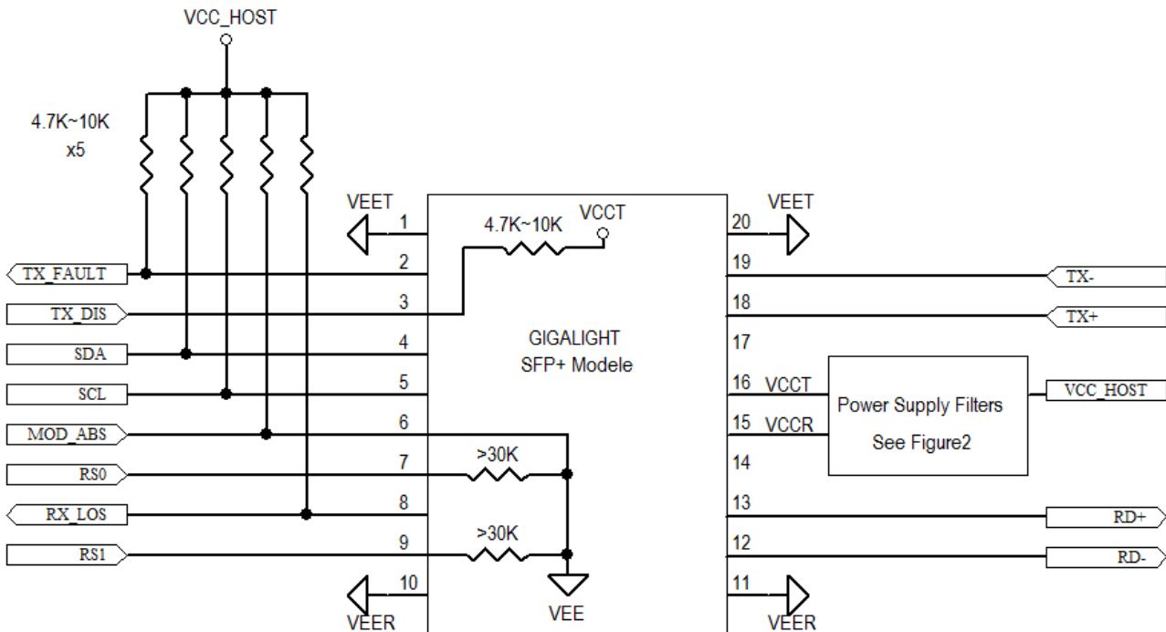
Рисунок 3. Host-Module Interface
