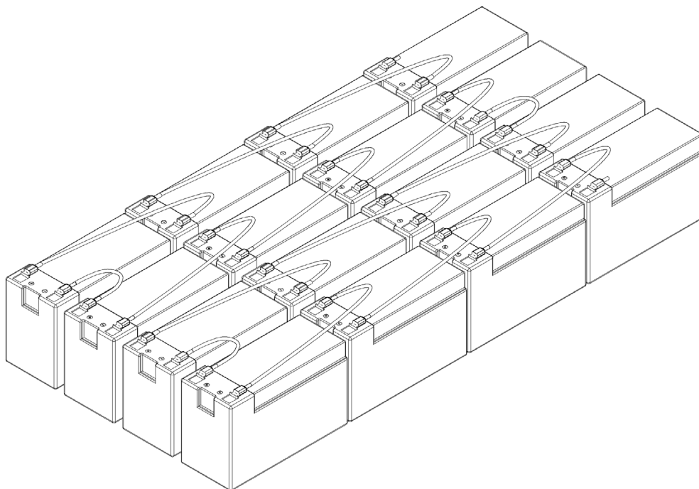
Рисунок 5 - Подключение АКБ в батарейном модуле
