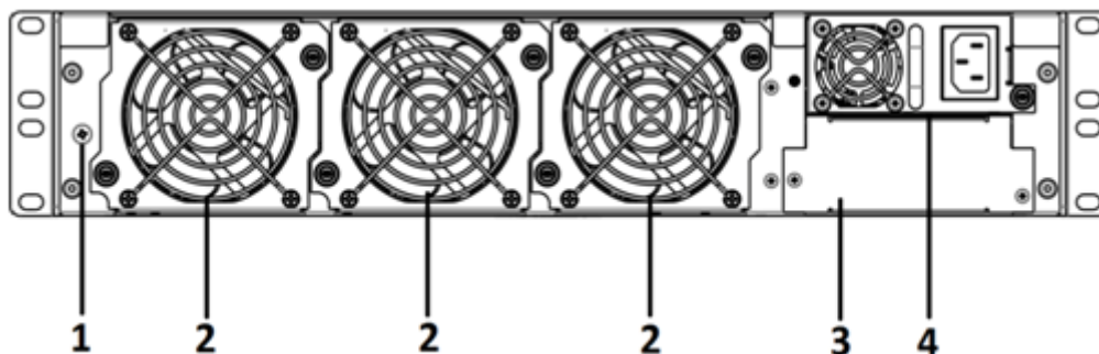
Рисунок 6 – Задняя панель ESR-1700
