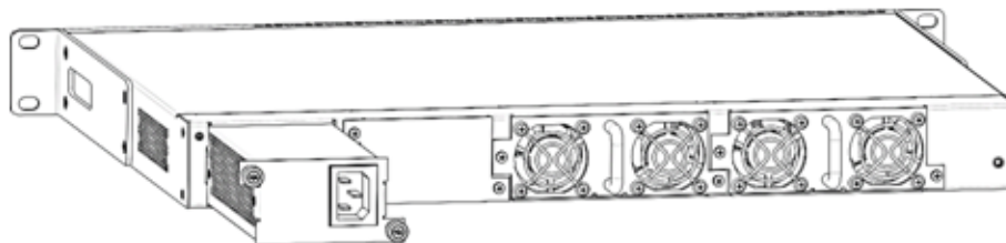
Рисунок 52 – Установка модулей питания
