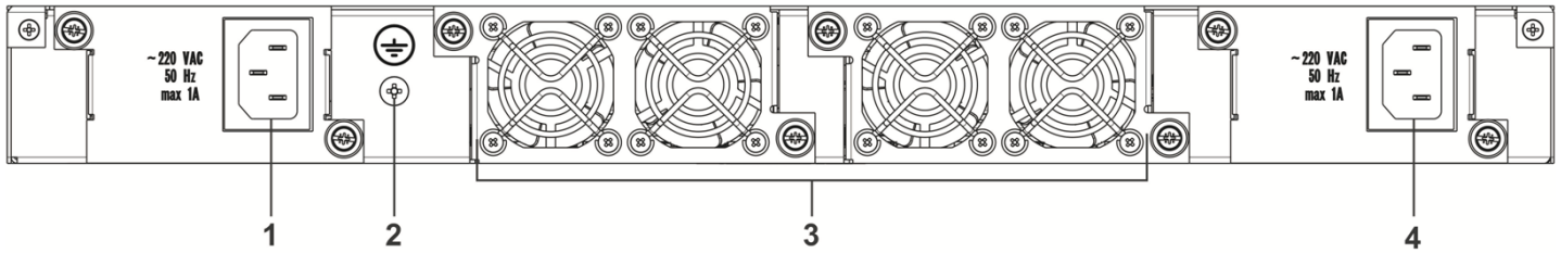
Рисунок 11 – Задняя панель ESR-1511, ESR-1500
