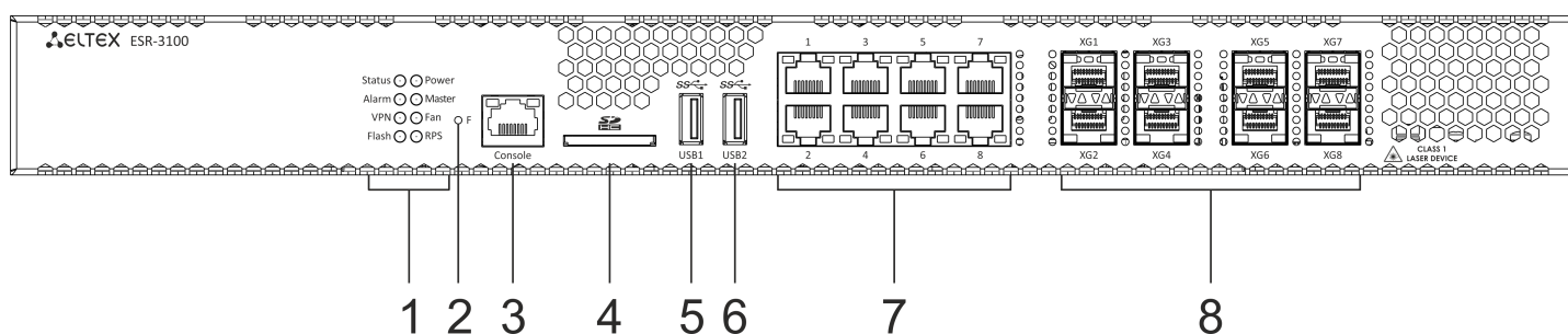
Рисунок 1 – Передняя панель ESR-3100
