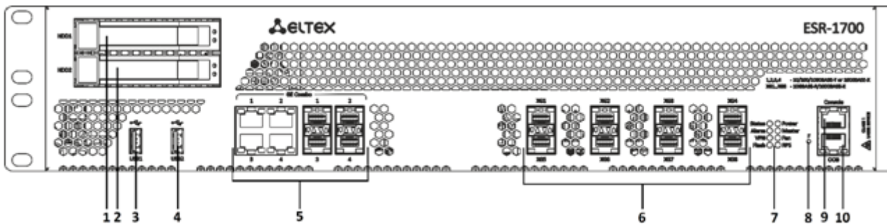
Рисунок 5 – Передняя панель ESR-1700
