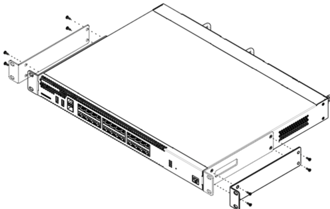
Рисунок 50 – Крепление кронштейнов
