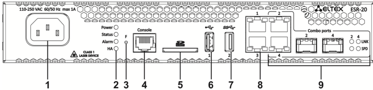
Рисунок 28 – Передняя панель ESR-20
