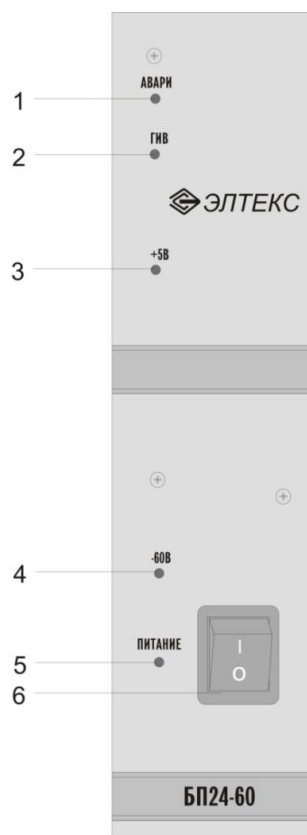
Рисунок 19 – Внешний вид панели БП24-60
