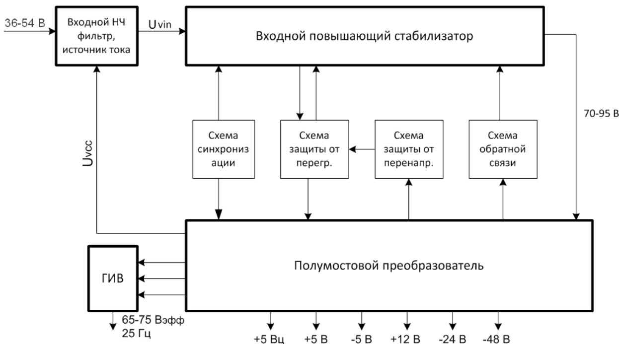
Рисунок 18 – Блок питания
