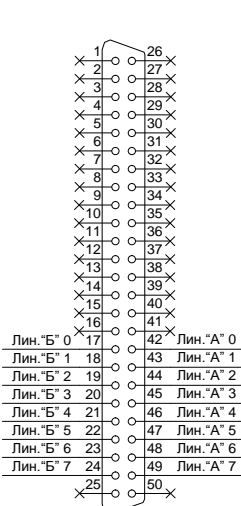
Модуль 16СК, 8АЛ
