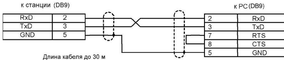
Схема кабеля для подключения к ПОРТ1, ПОРТ2
