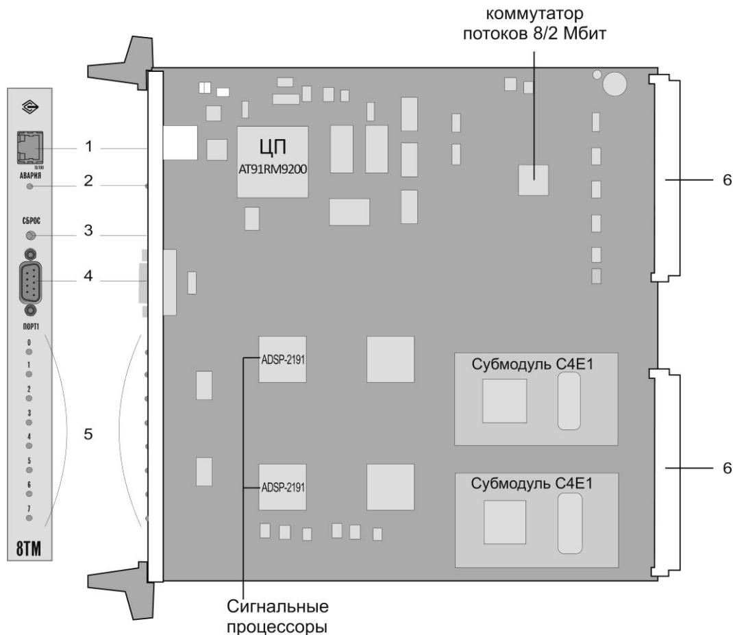
Рисунок 14 – Внешний вид панели и платы модуля 8ТМ
