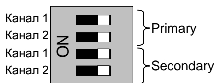
Рисунок 13 – DIP-переключатели
