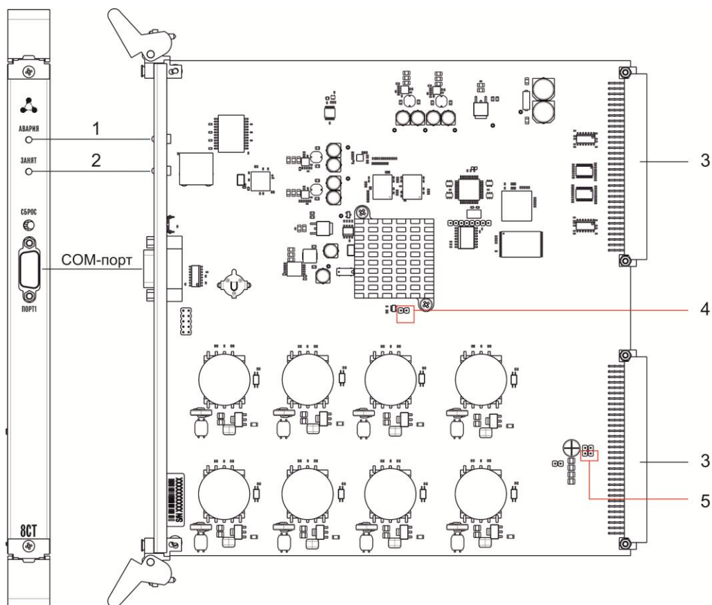
Рисунок 9 – Внешний вид панели и платы модуля 8СТ
