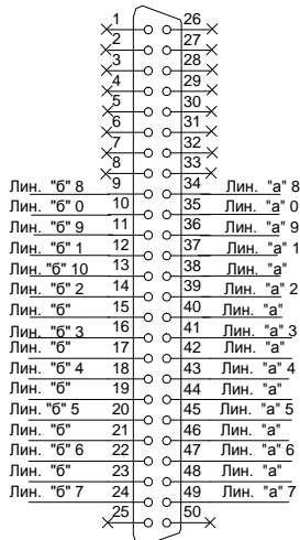
Модуль 16СТ, 8СТ (Лин. 0...7)
