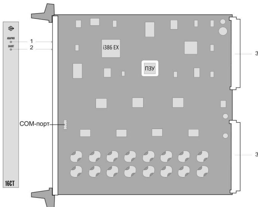
Рисунок 8 – Внешний вид панели и платы модуля 16СТ
