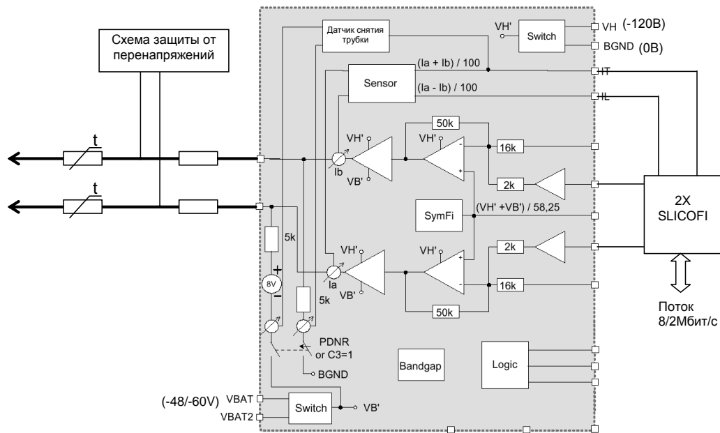
Рисунок 7 – Упрощенная принципиальная схема одного 24АК (24АК-Д)
